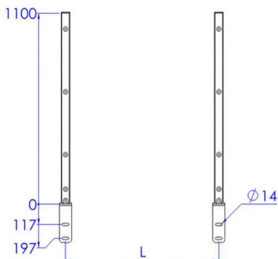
Potelets avec garde-corps | Top fixing with guardrail
